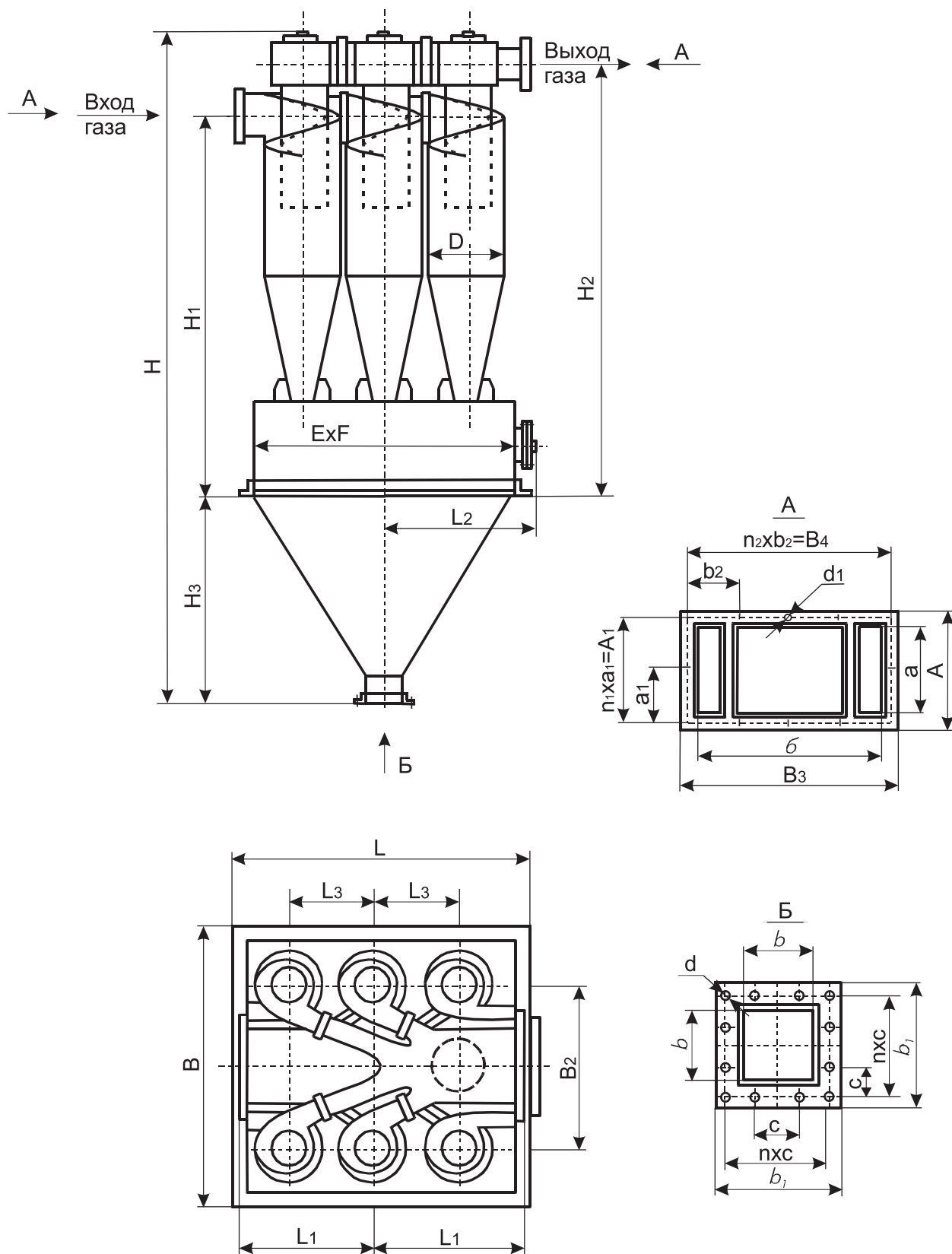
Рис.4 Циклон типа ЦН-15х6УП.
