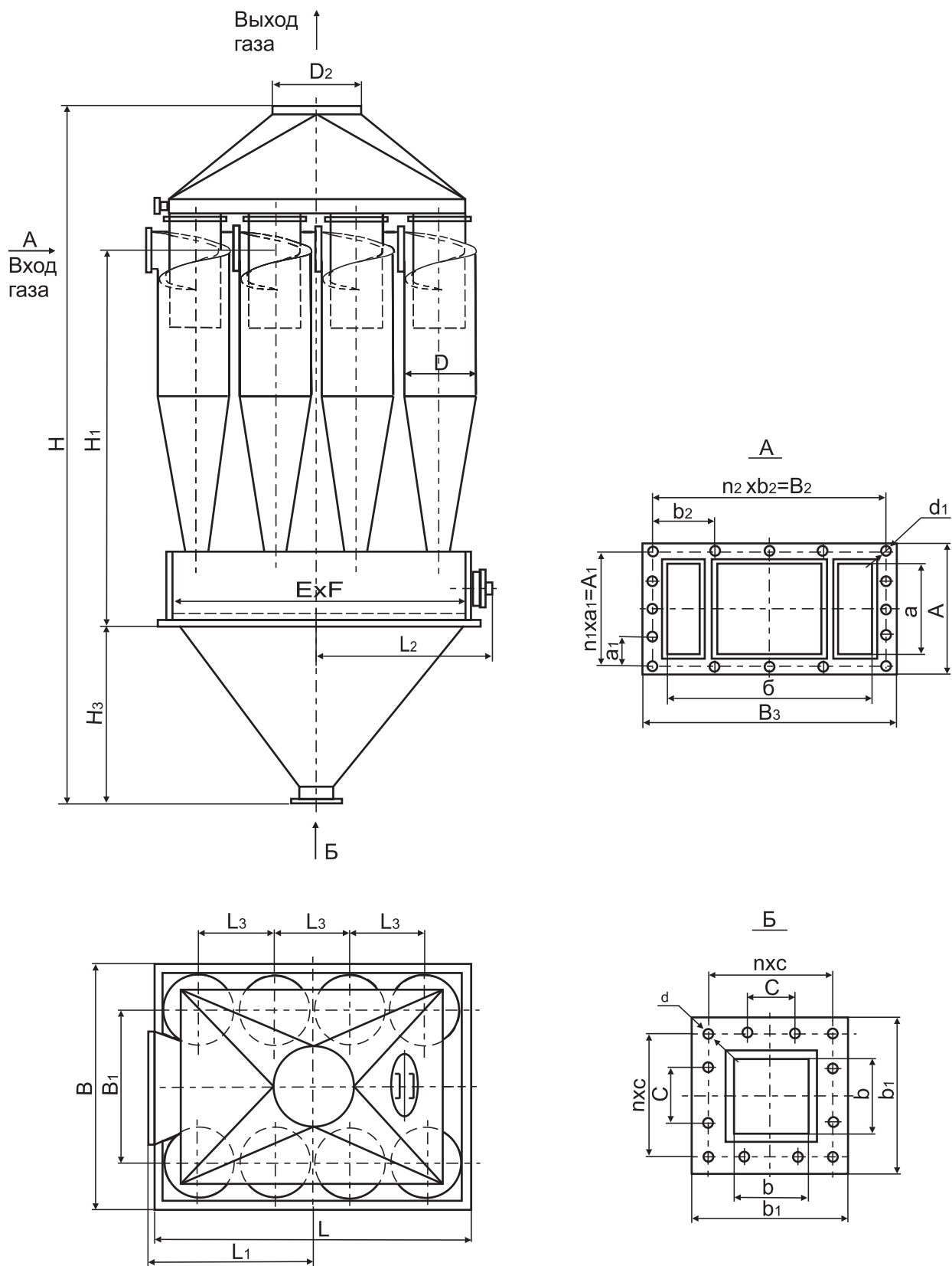
Рис.8 Циклон типа ЦН-15х4СП.
