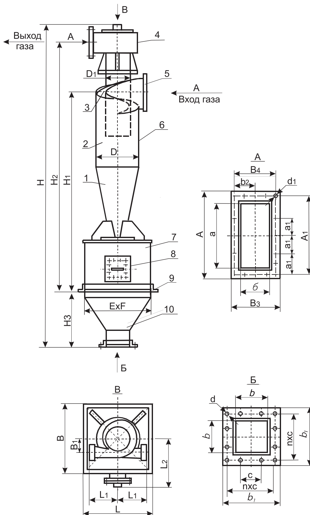
Рис.1 Циклон типа ЦН-15х1УП
