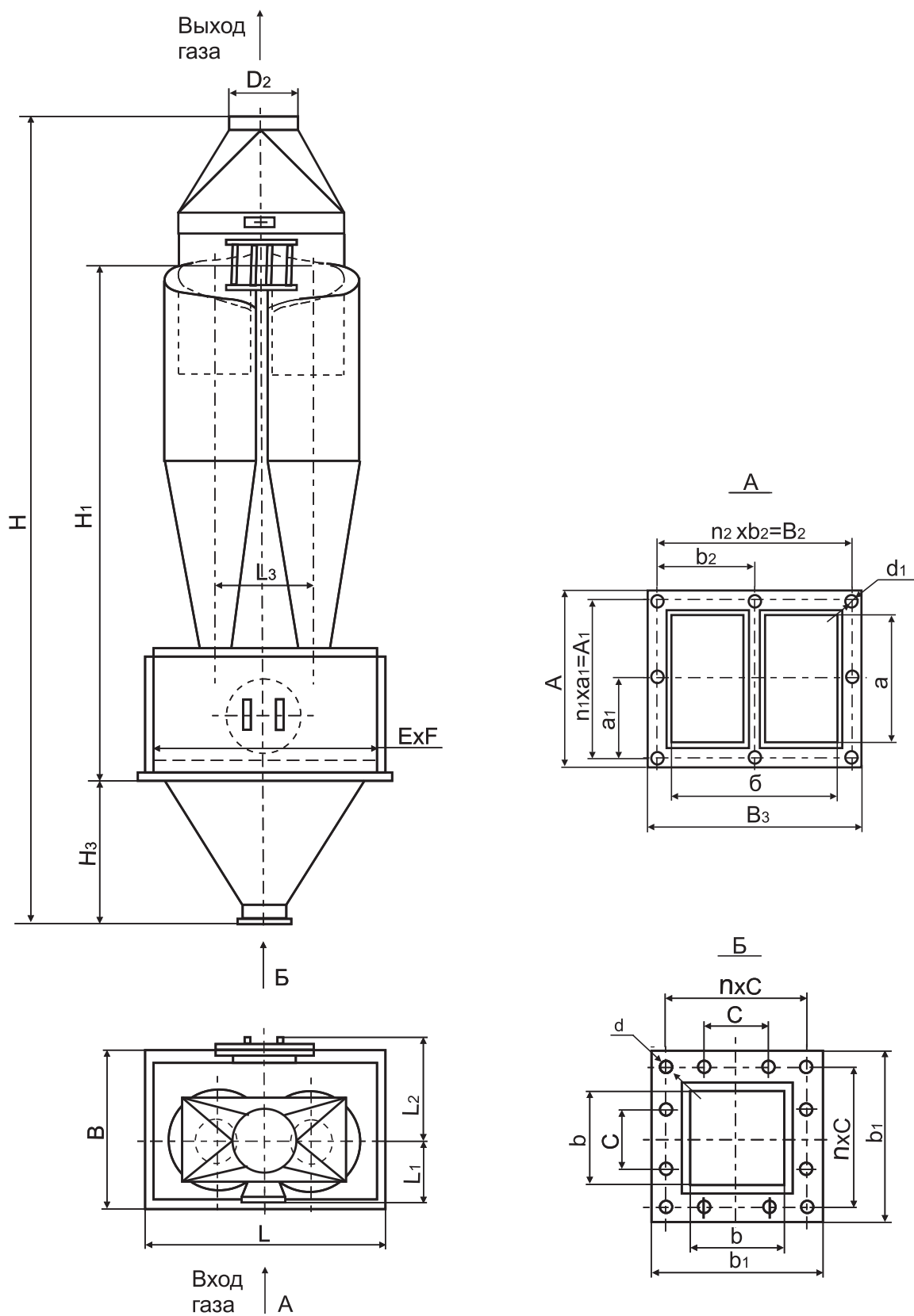
Рис.5 Циклон типа ЦН-15х2СП.
