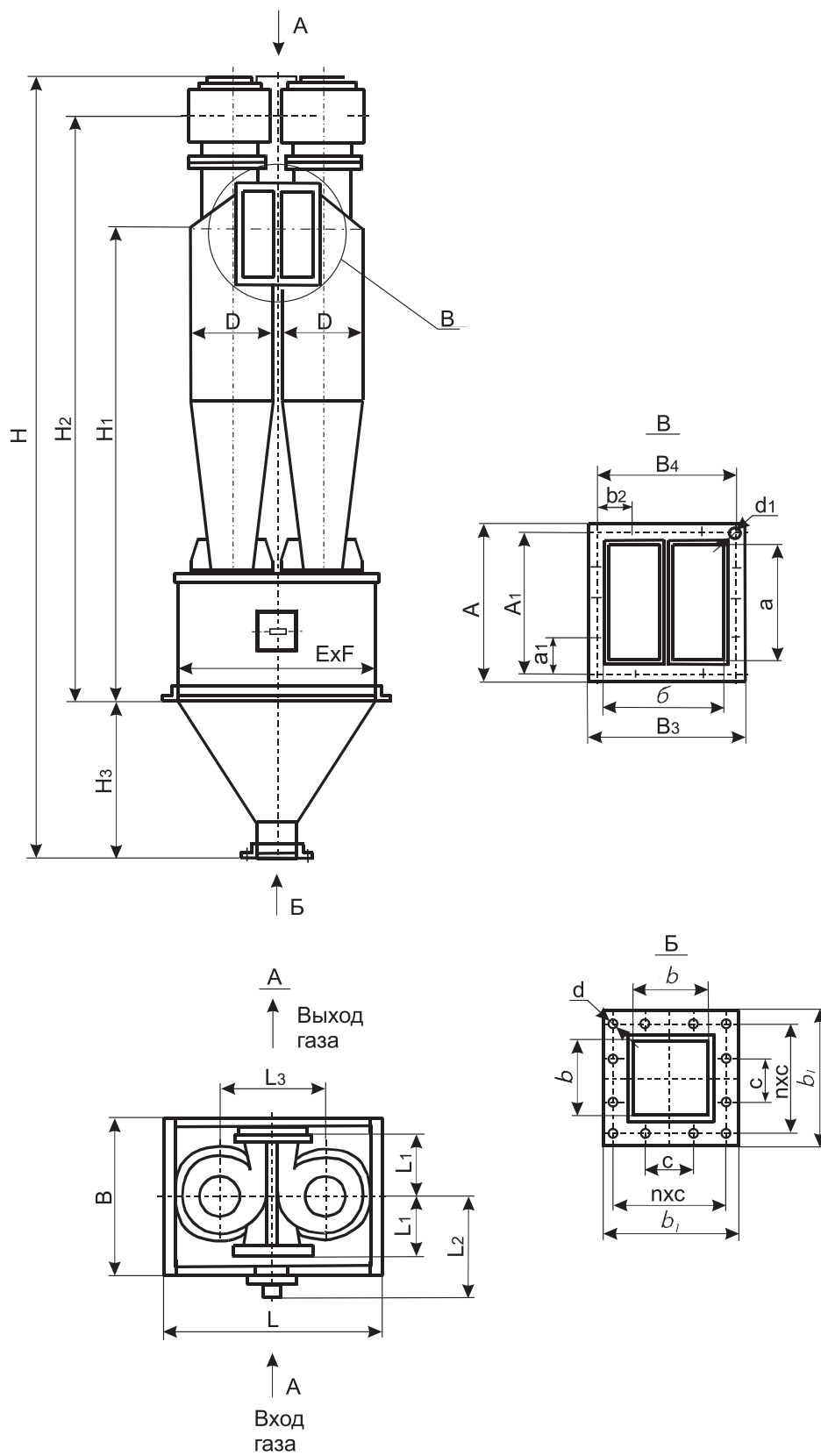
Рис.2 Циклон типа ЦН-15х2УП.
