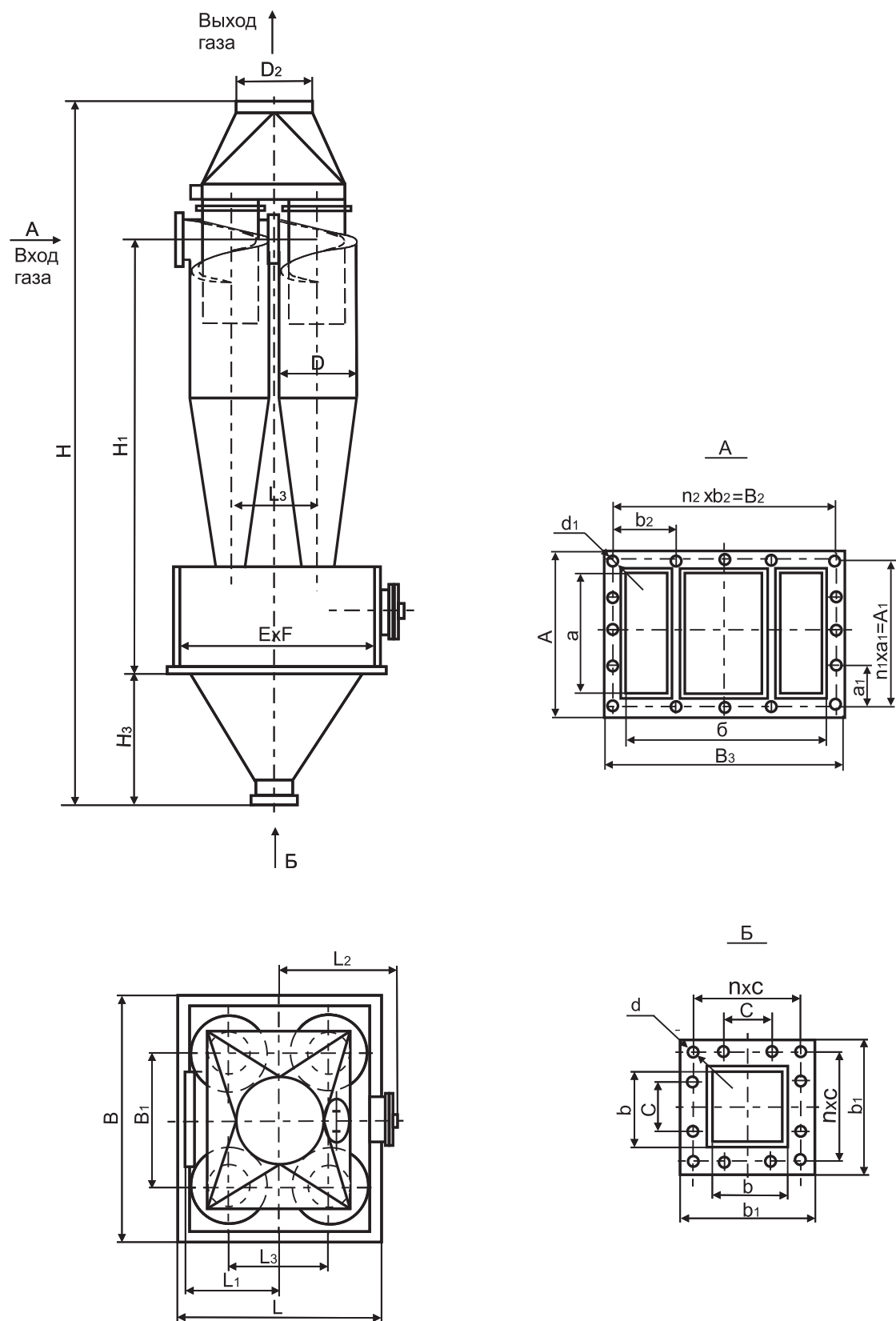
Рис.6 Циклон типа ЦН-15х4СП.
