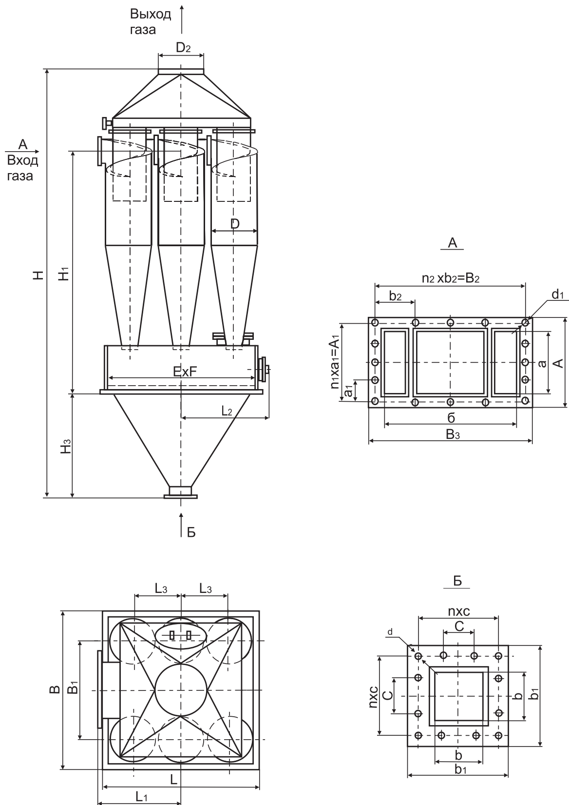
Рис.7 Циклон типа ЦН-15х6СП.
