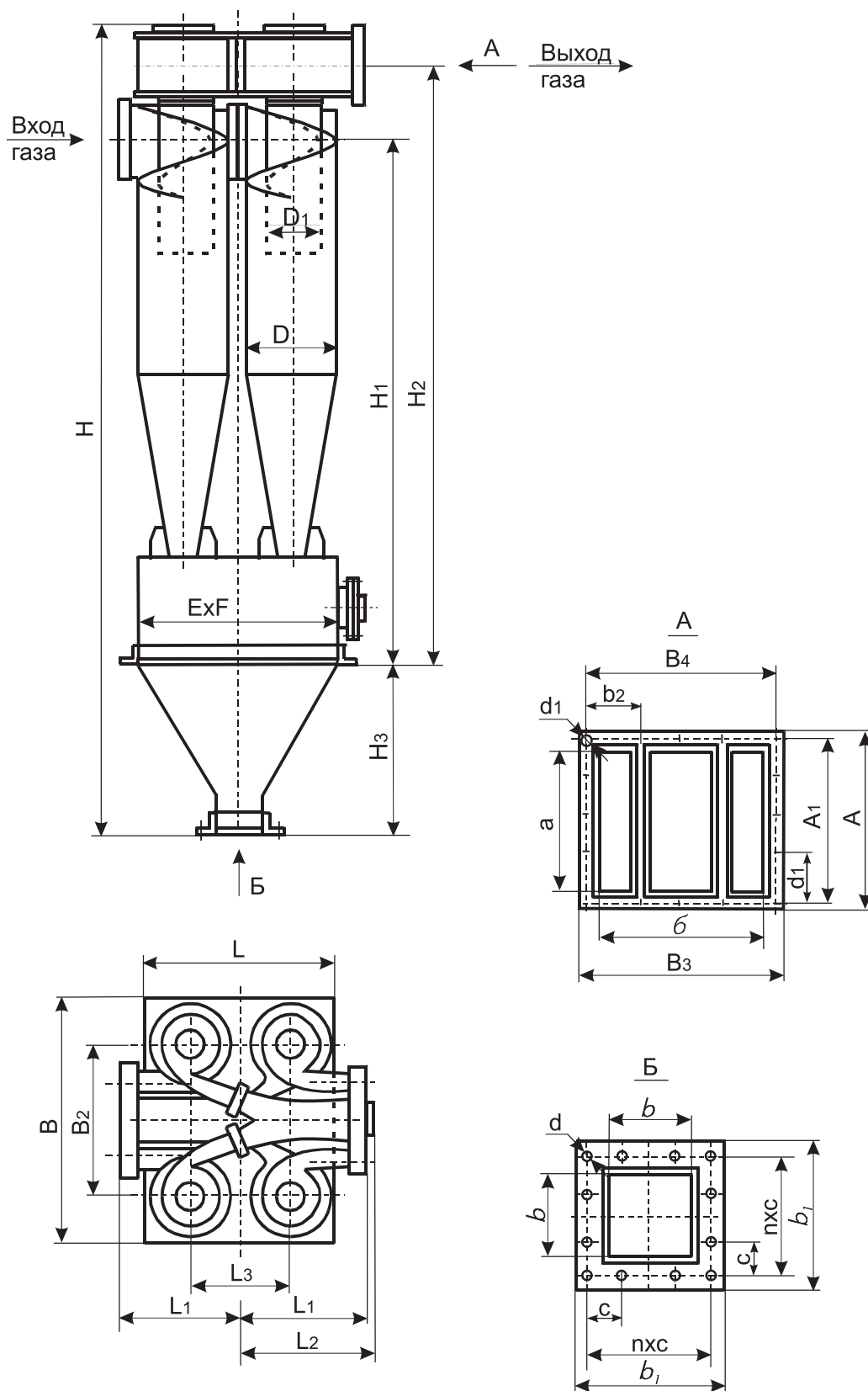
Рис.3 Циклон типа ЦН-15х4УП.
